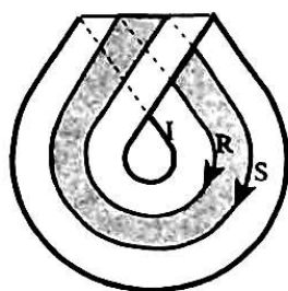
Double tour dans le plan projectif avec R Bande de Mœbius dans la bande de Mœbius
