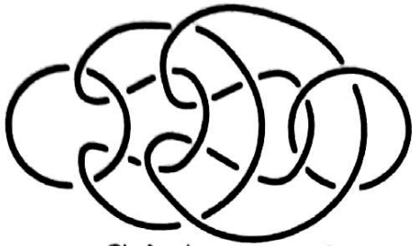
Chaîne à quatre avec S
