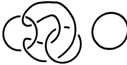
Chaîne à trois : S glisse
