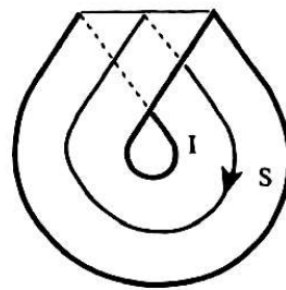
Tour simple dans le plan projectif R rétracté Coupure dans la bande de Mœbius
